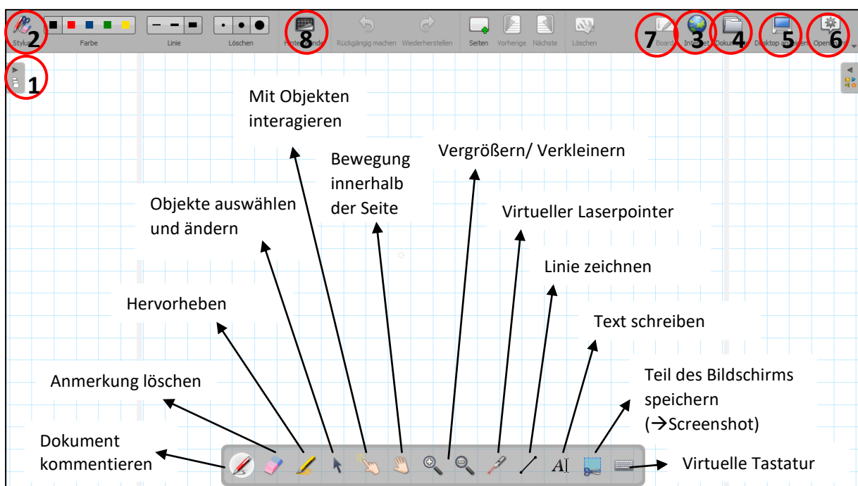
Abbildung 1: Startbildschirm OpenBoard
